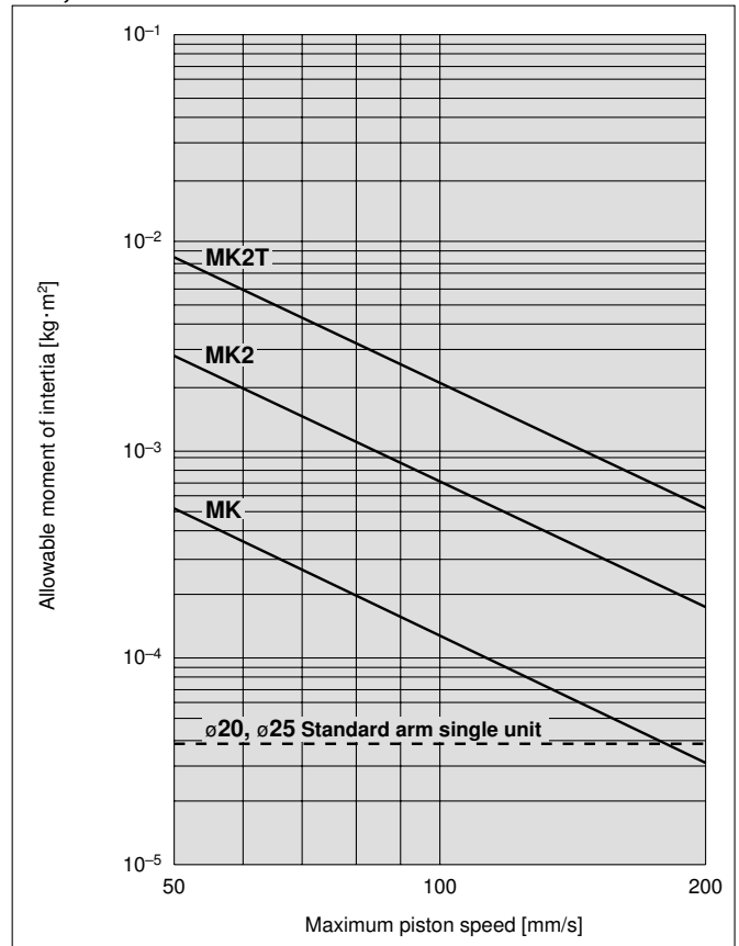
ø50, ø63
