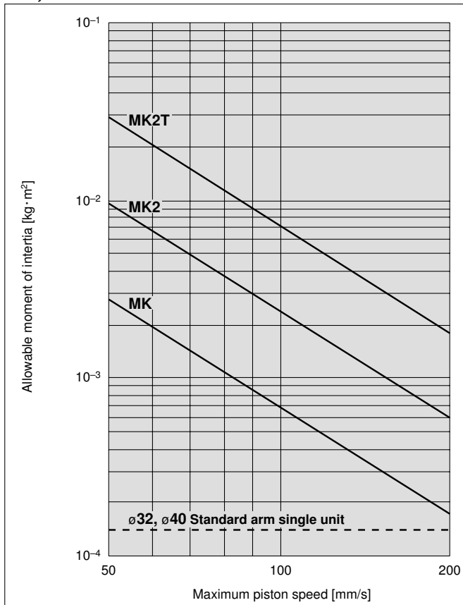
ø32, ø40
